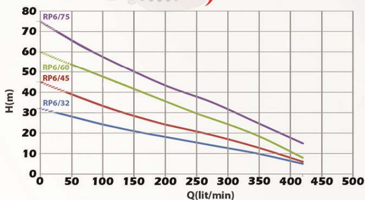
2" inch منحني میزان آبدهی - ارتفاع H(m)
