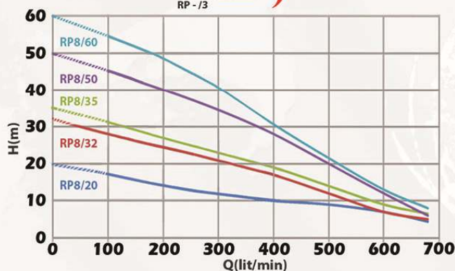
3" inch منحني میزان آبدهی - ارتفاع H(m)
